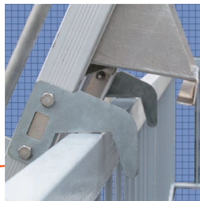
型枠の上側に固定できるフックがついています。
