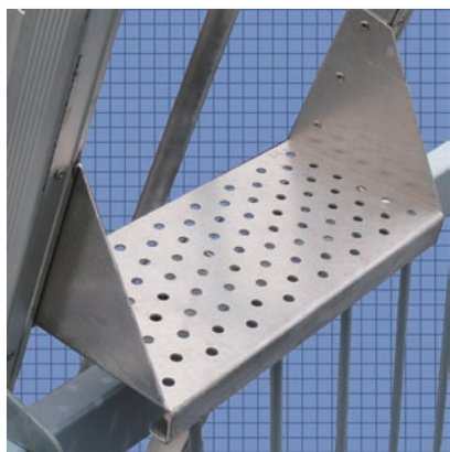
最上段のステップ幅が広く安全です
