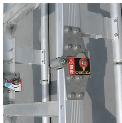
自動ロック式折畳み金具
